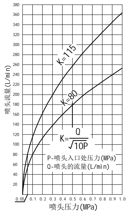
压力与流量关系曲线
