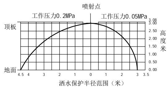
ZSTKZ20直立型喷头喷射曲线
