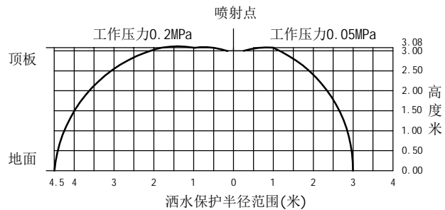
ZSTKZ20直立型喷头喷射曲线
