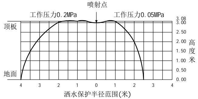
ZSTKZ15直立型喷头喷射曲线
