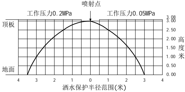
ZSTKX15下垂型喷头喷射曲线
